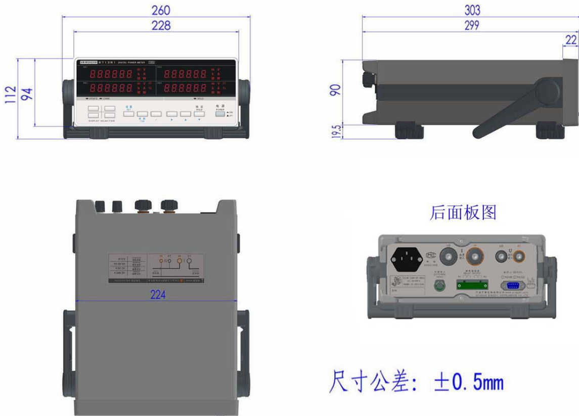
图 1 外形尺寸图
